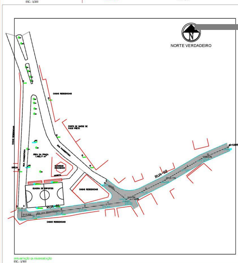
IMPLANTAÇÃO DA PAVIMENTAÇÃO ESC.: 1/500
