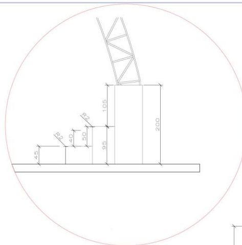
VISTA DA ARQUIBANCADA
