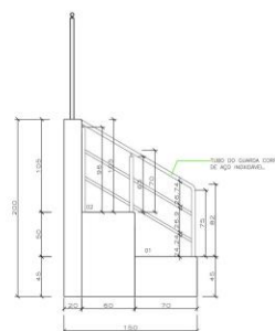
VISTA LATERAL DA ARQUIBANCADA Esc. 1:25
