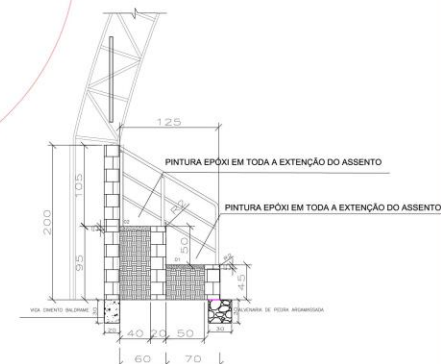
CORTE TRANSVERSAL ARQUIBANCADA
